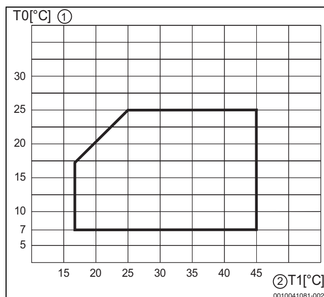
Fig. 5 Pompe à chaleur en mode Refroidissement
