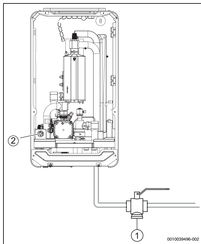
Fig. 13 Unité intérieure Compress 5800i 12 E
