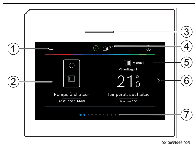
Fig. 8 Tableau de commande
