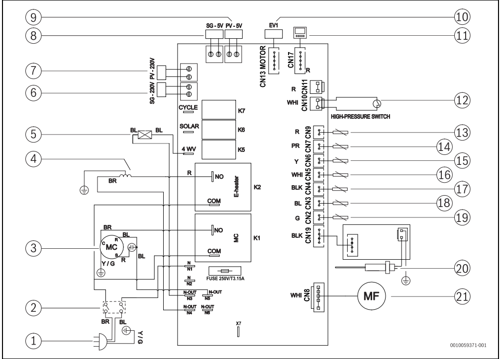
Fig. 33 Schéma électrique
