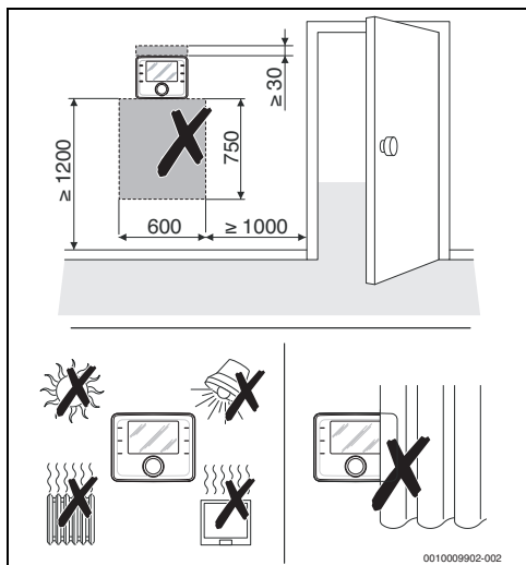
Fig. 5 Lieu d'installation dans la pièce de référence
