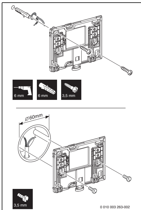
Fig. 6 Montage du socle
