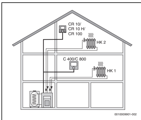
Fig. 2 CR 10/CR 10 H/CR 100 en tant que commande à distance pour le deuxième circuit de chauffage (HK 2) et C 400/C 800 en tant qu'appareil de régulation pour le premier circuit de chauffage (HK 1)
